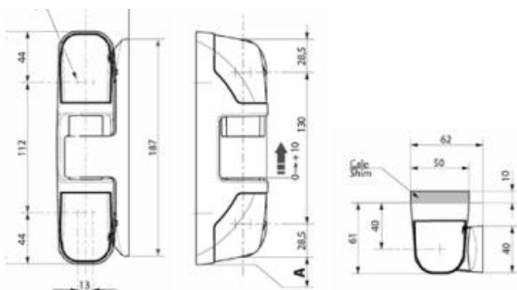
Charnière 1472 sans rampe
