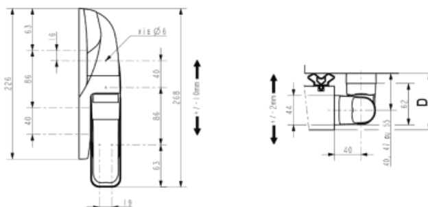
Charnière 1573 décalage huisserie 40
